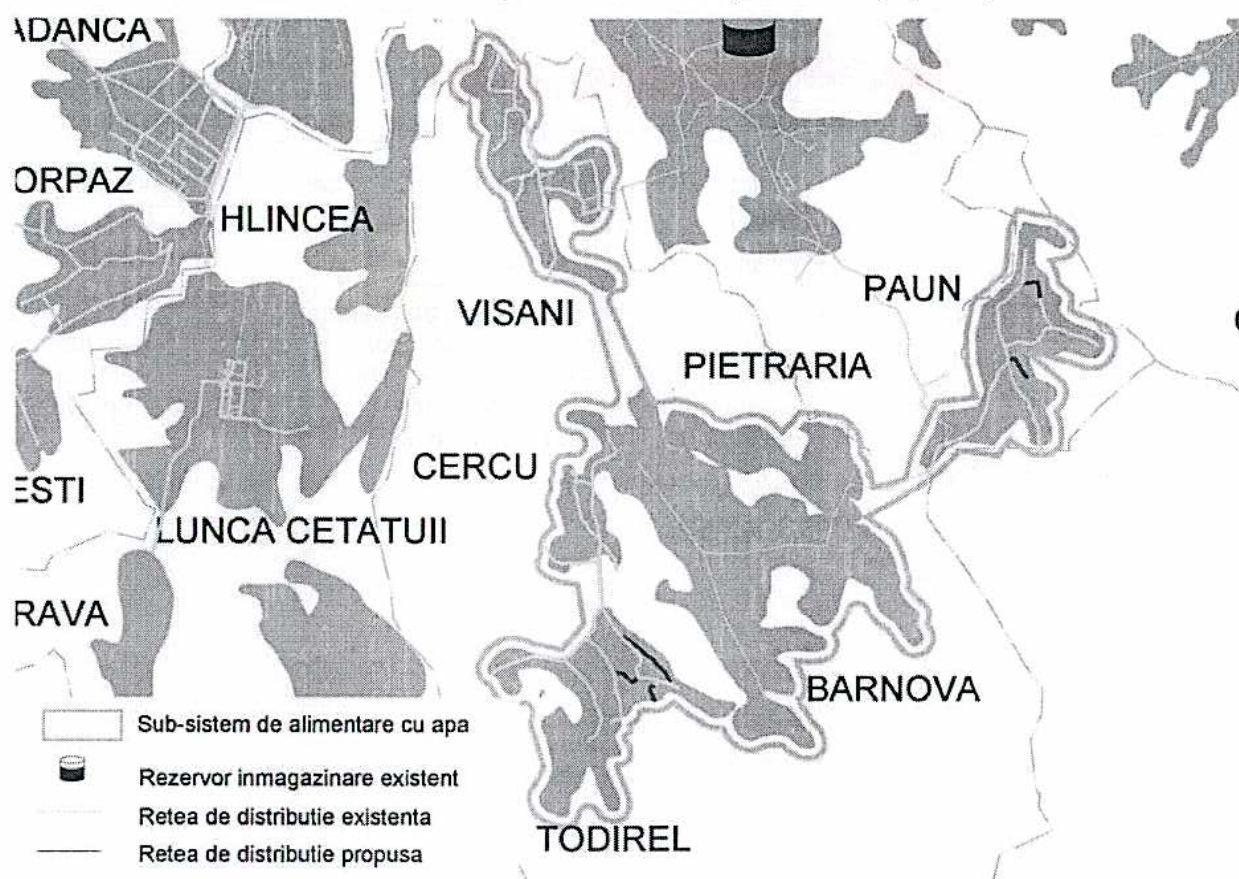
Figura 9-21 - Sub-sistemul de alimentare cu apa Barnova
